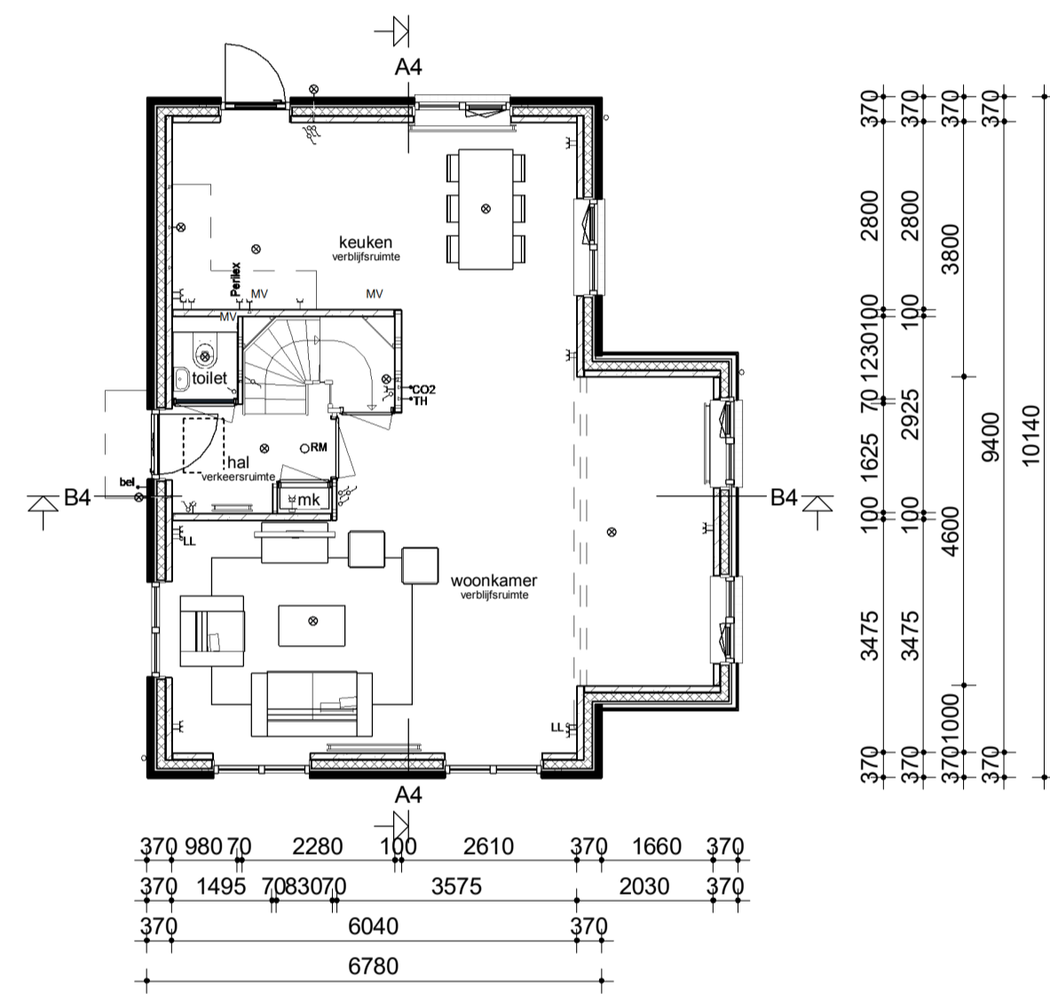
Begane grond
