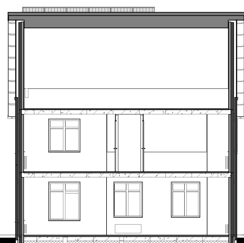
Doorsnede A4
