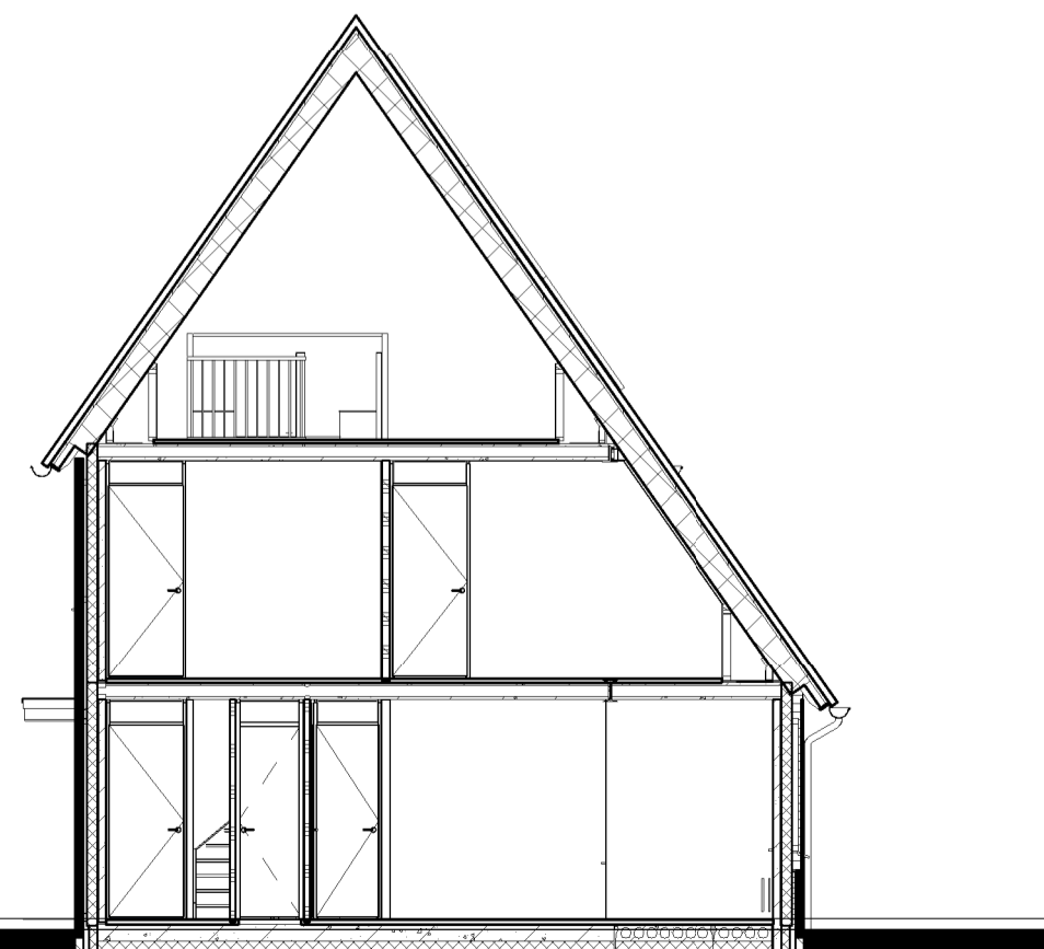
Doorsnede B4
