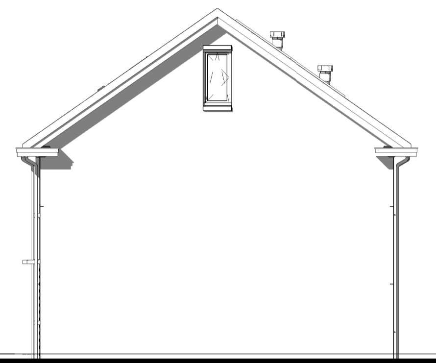
Rechter zijgevel
