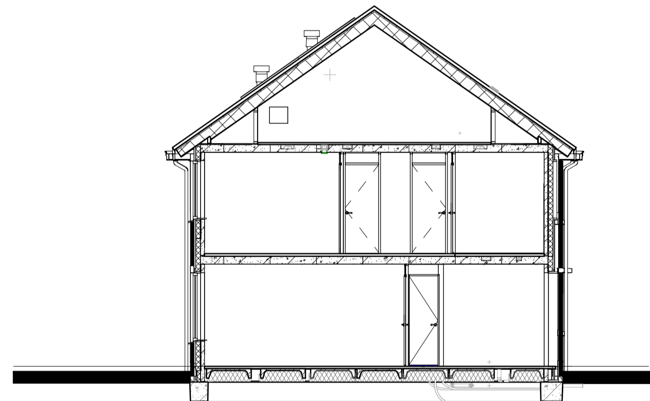
Doorsnede A1-A1
