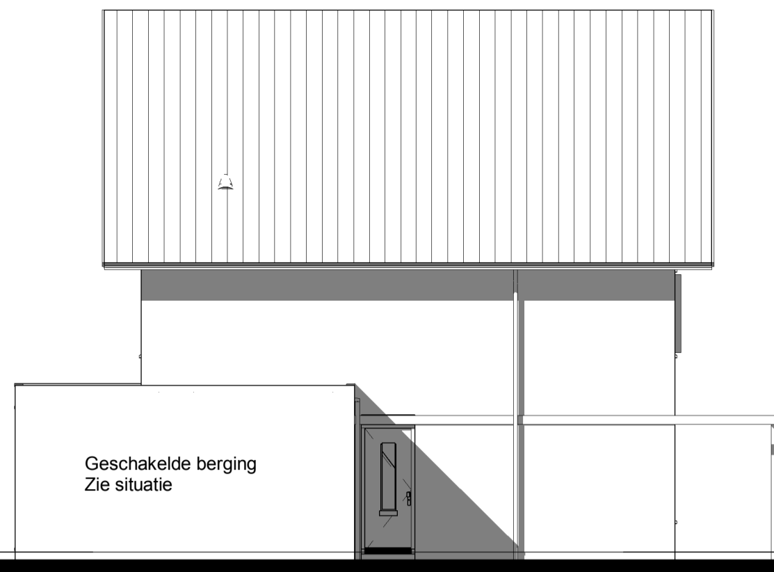
Linker zijgevel
