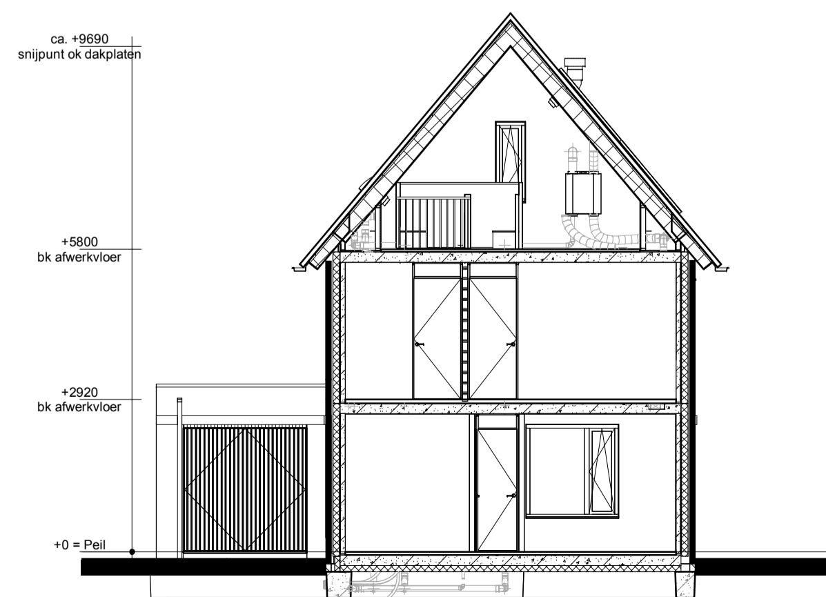
Doorsnede B1
