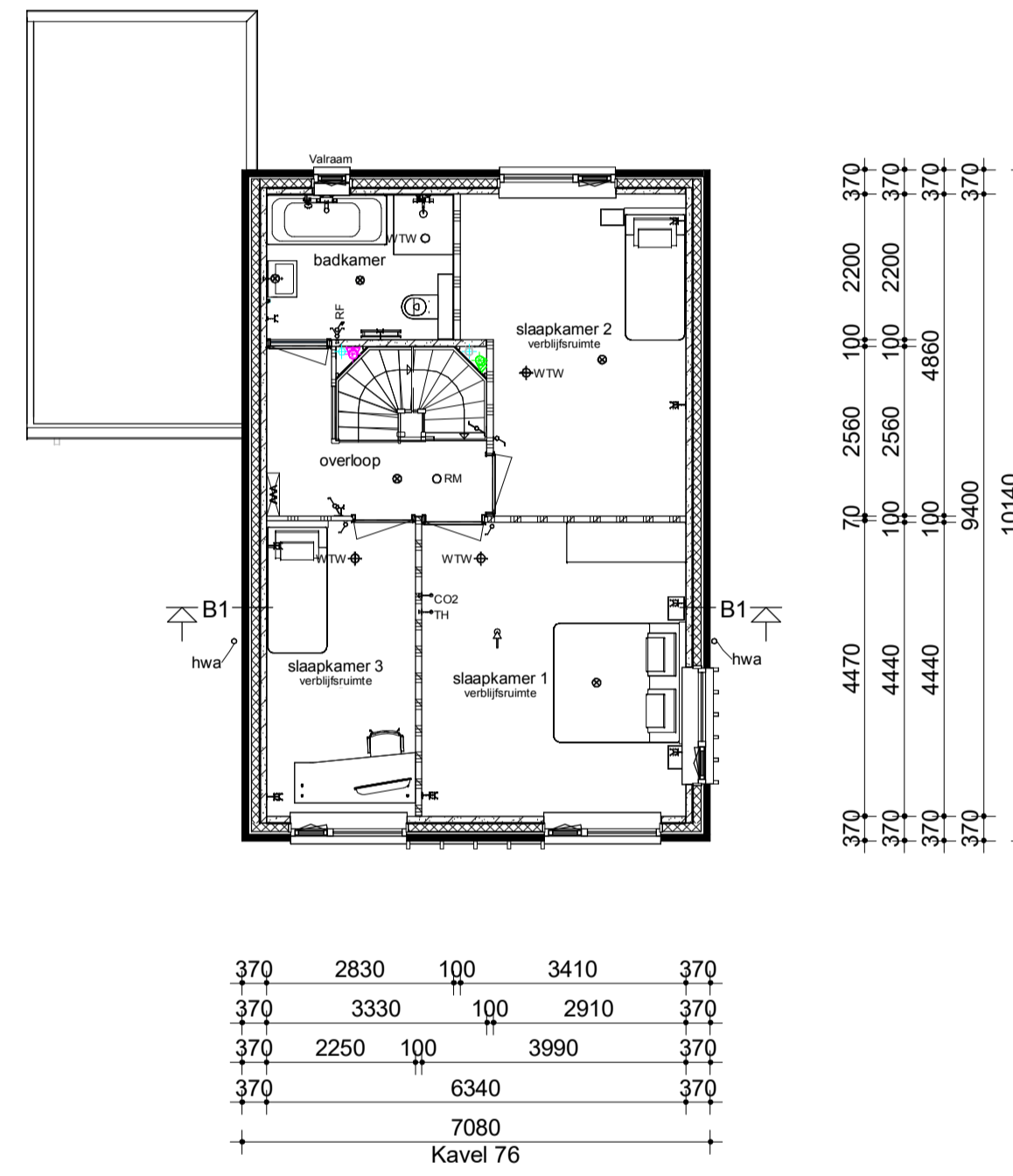
Verdieping
