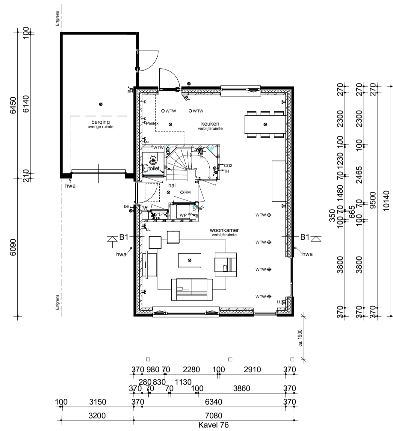
Begane grond
