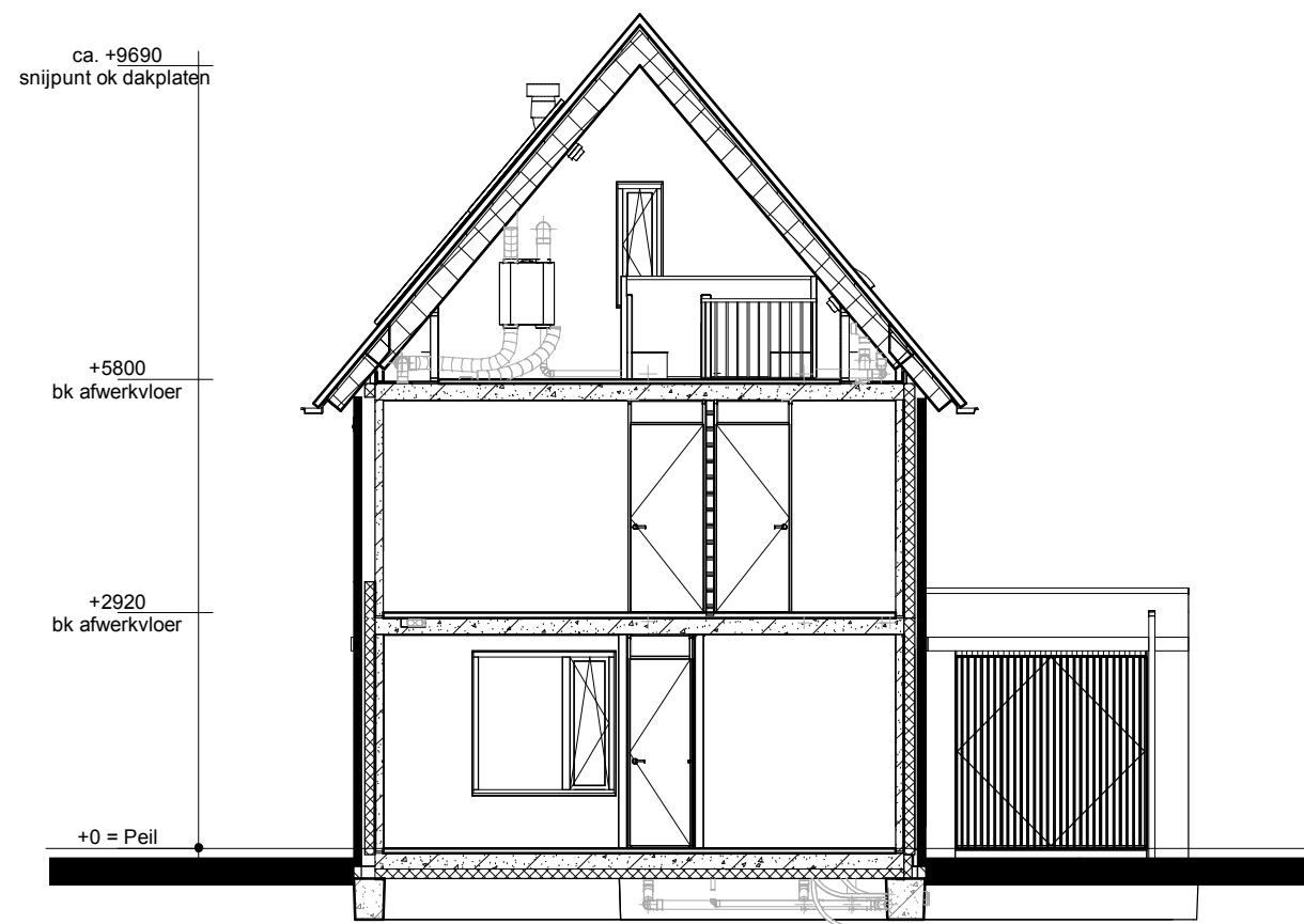
Doorsnede B5
