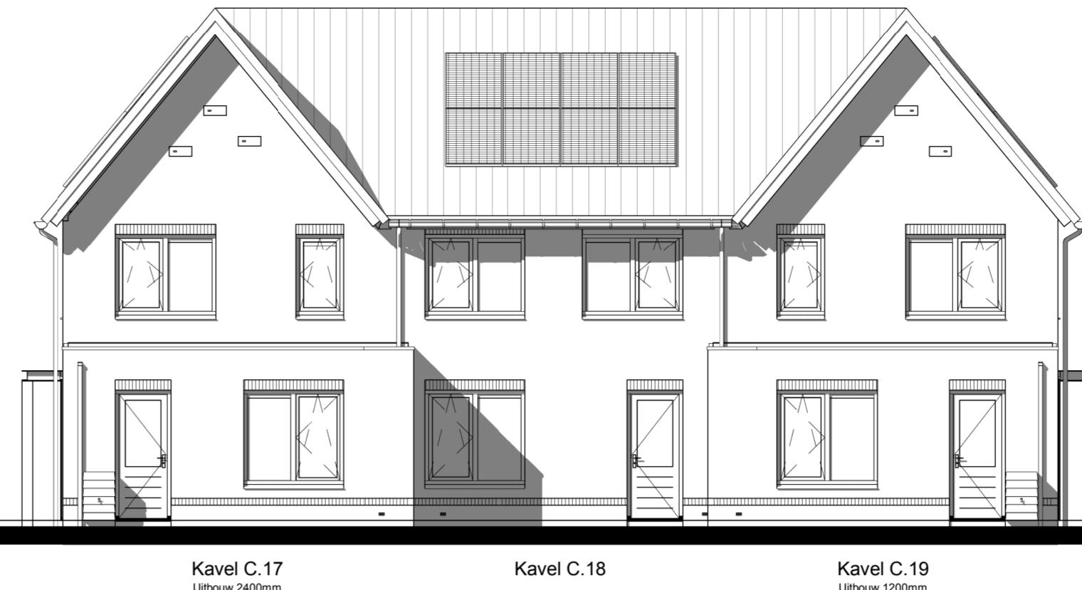
Achtergevel
