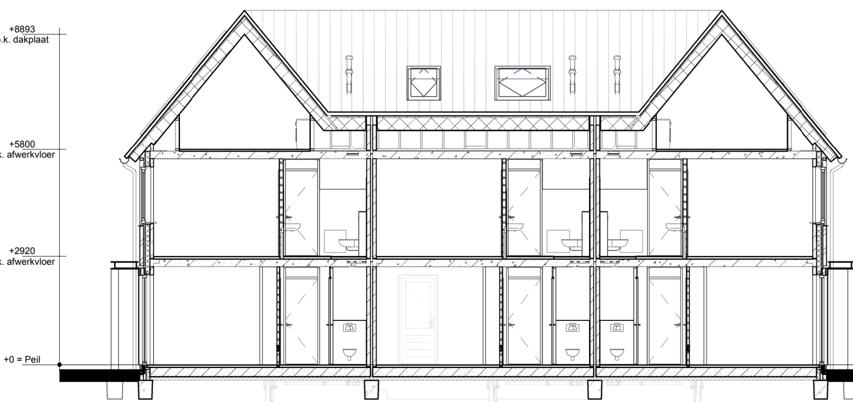
Doorsnede B-B
