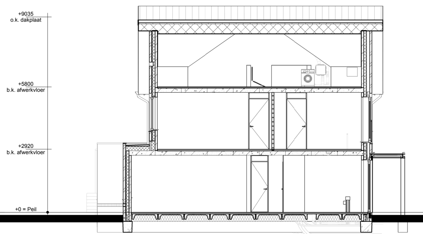
Doorsnede A-A
