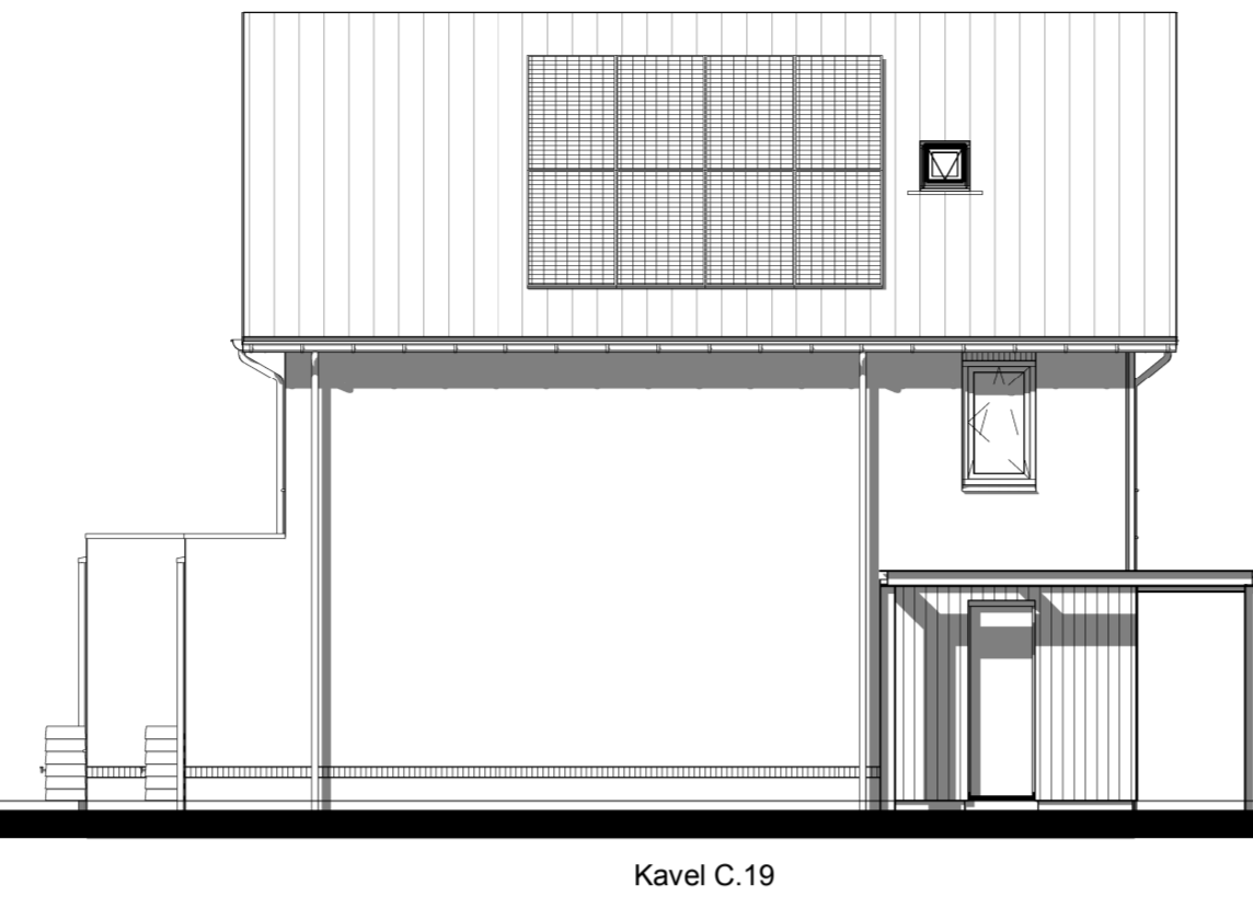
Linker zijgevel
