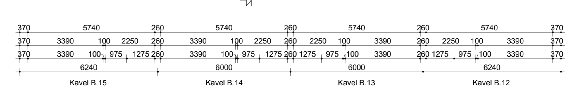
Verdieping
