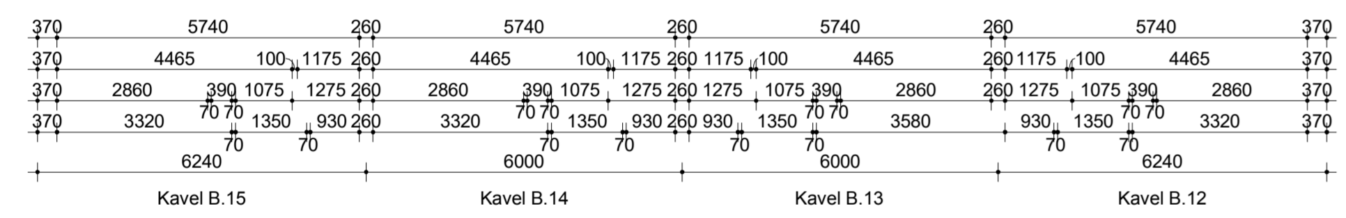
Begane grond
