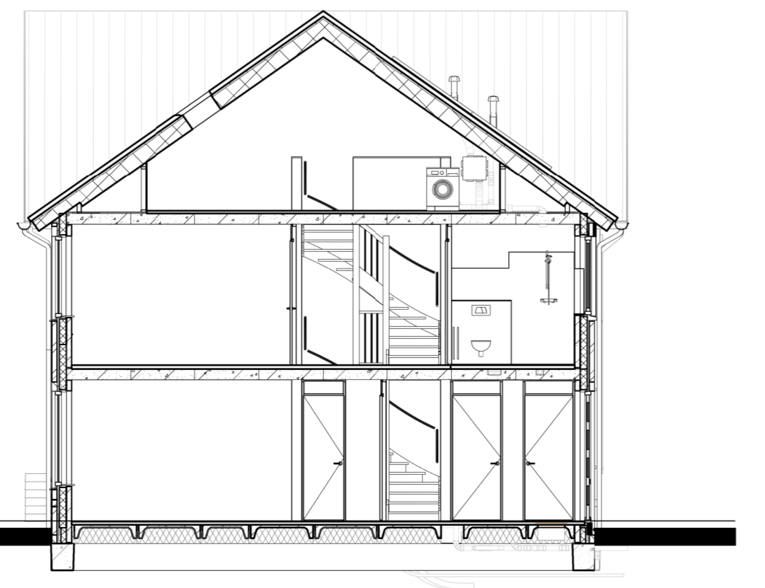
Doorsnede A-A
