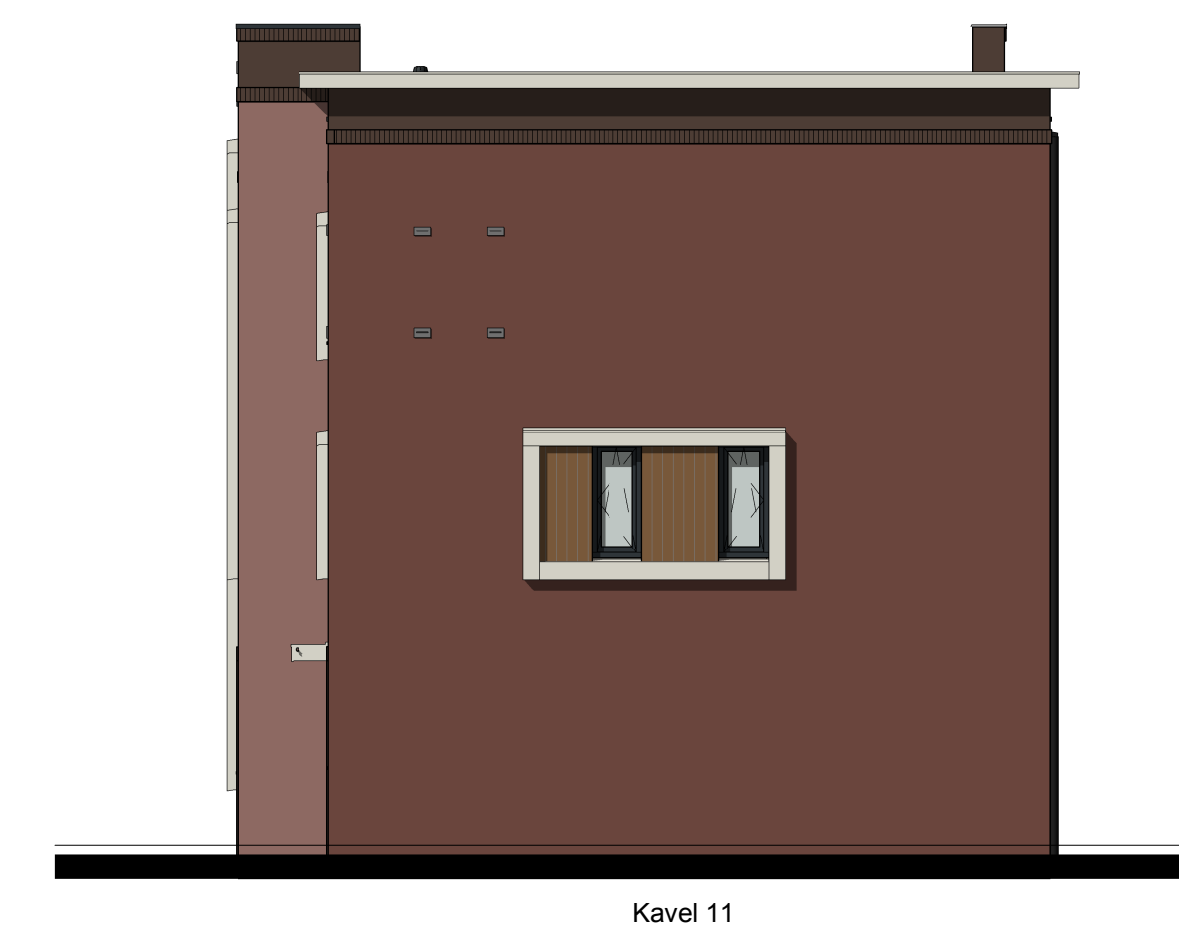
Rechter zijgevel
