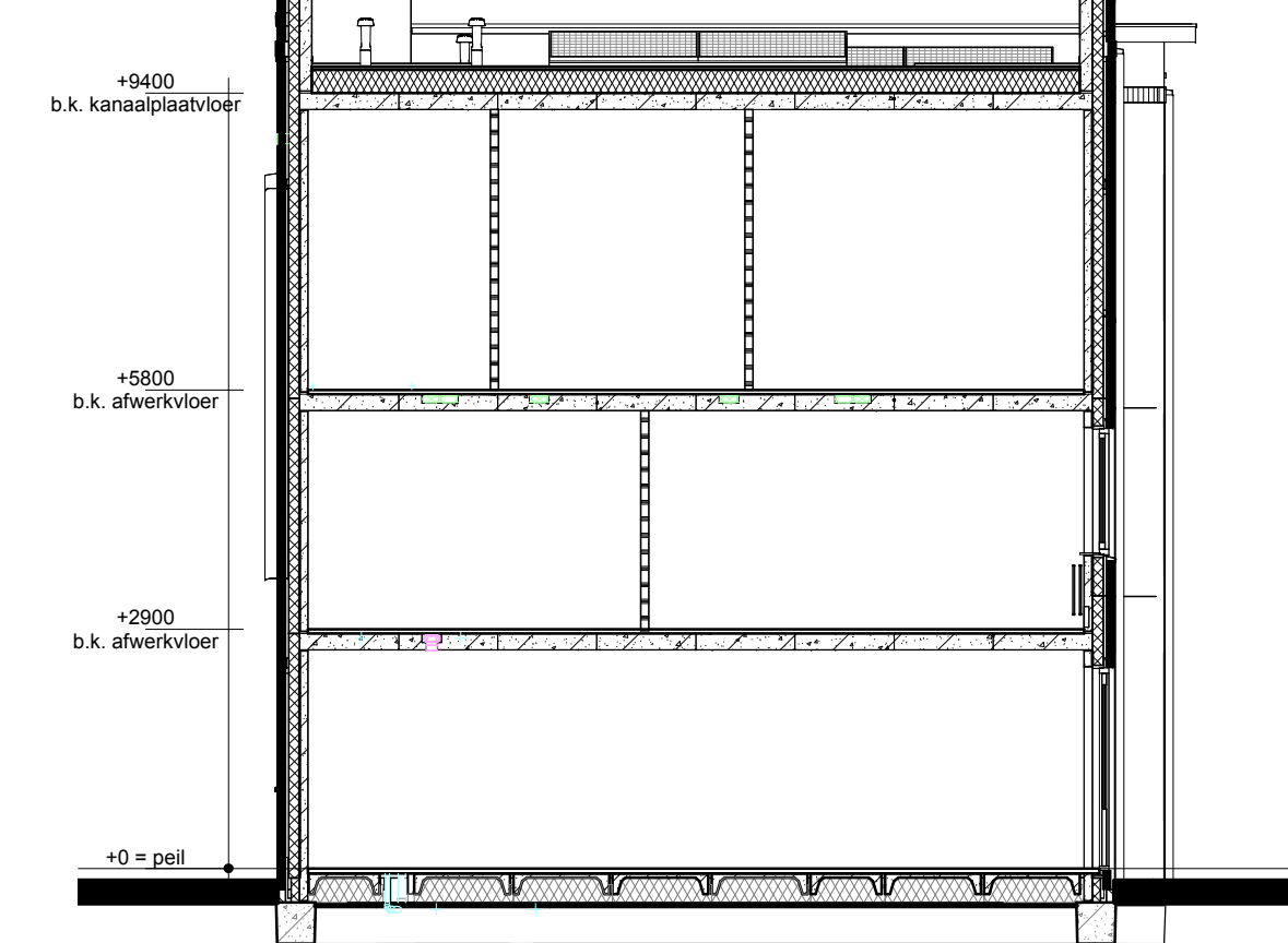
Doorsnede A2-A2
