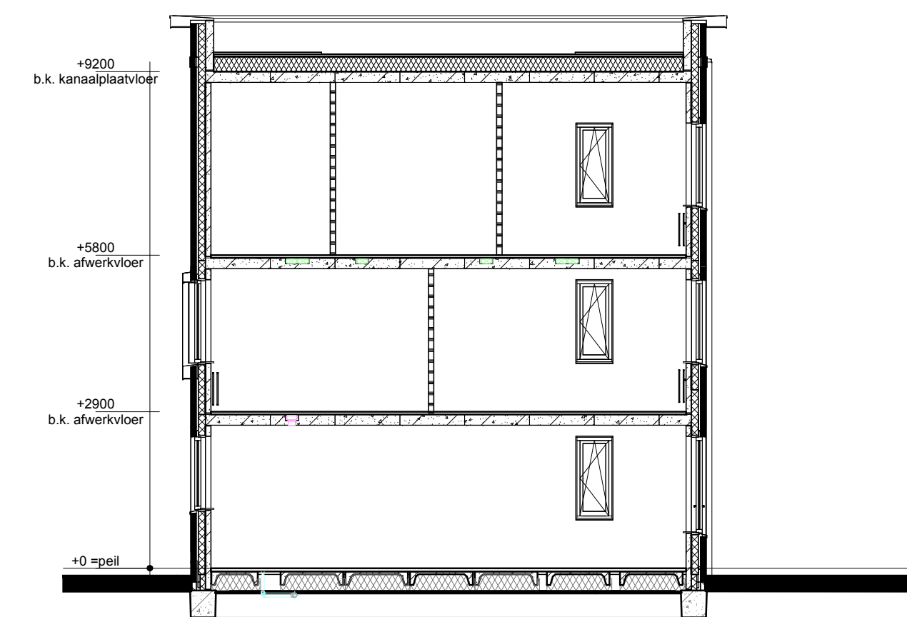
Doorsnede A1-A1
