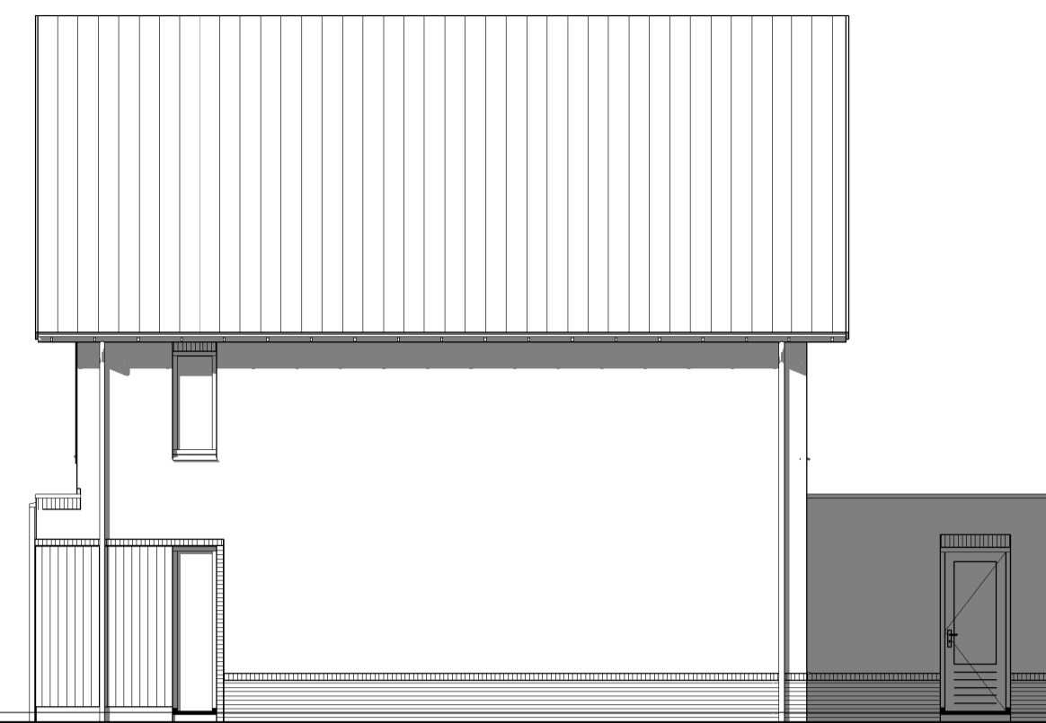
Rechter zijgevel
