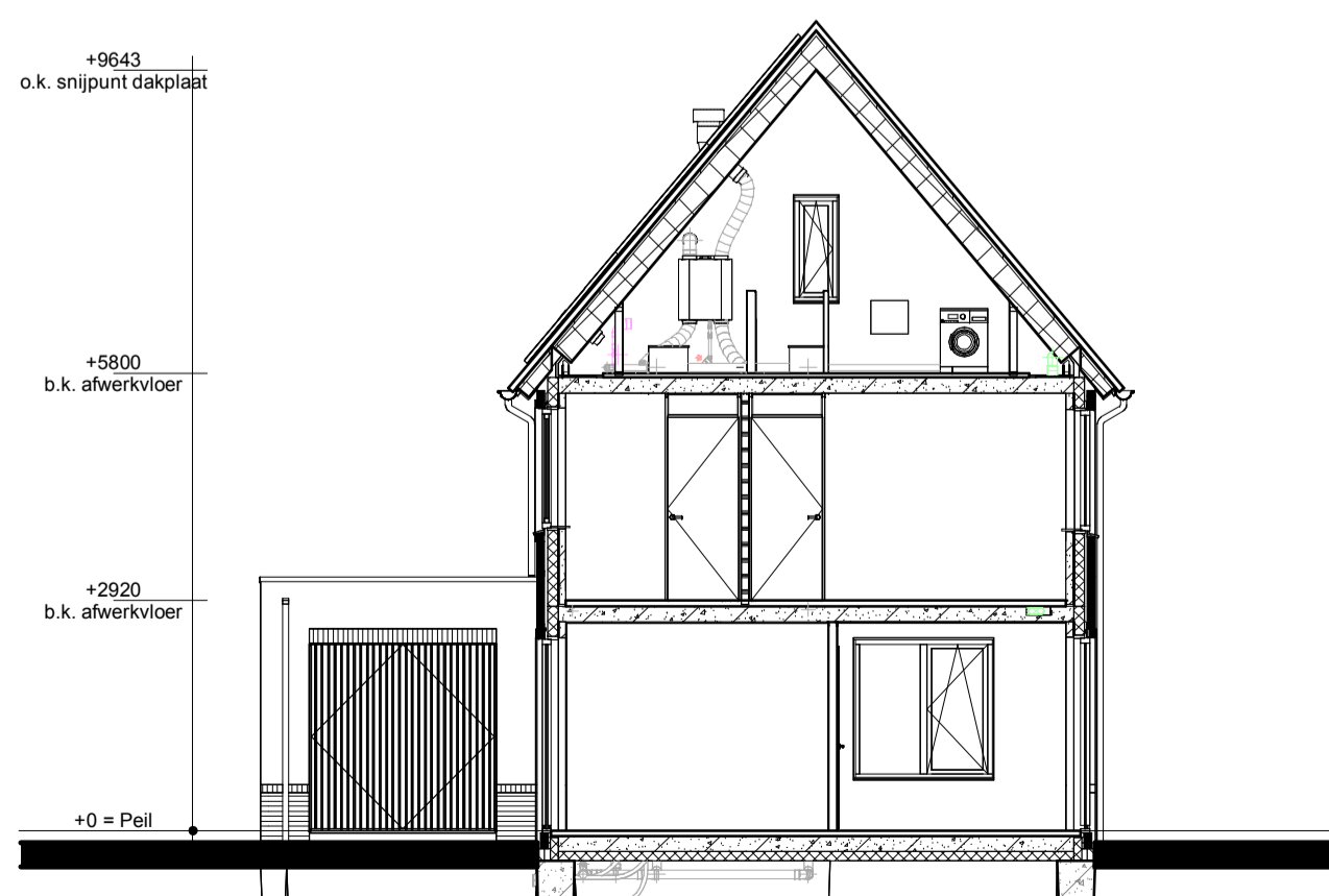
Doorsnede B1-B1
