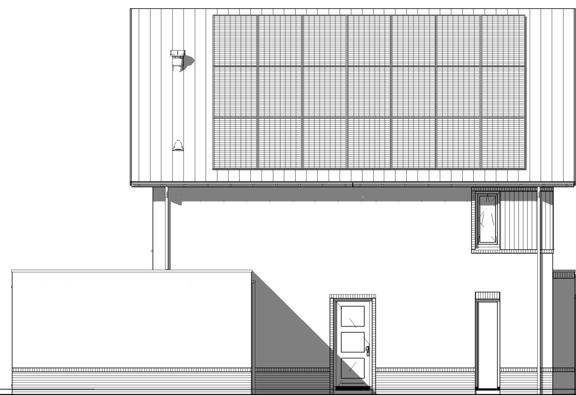
Linker zijgevel
