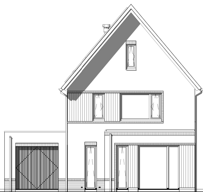
Voorgevel
