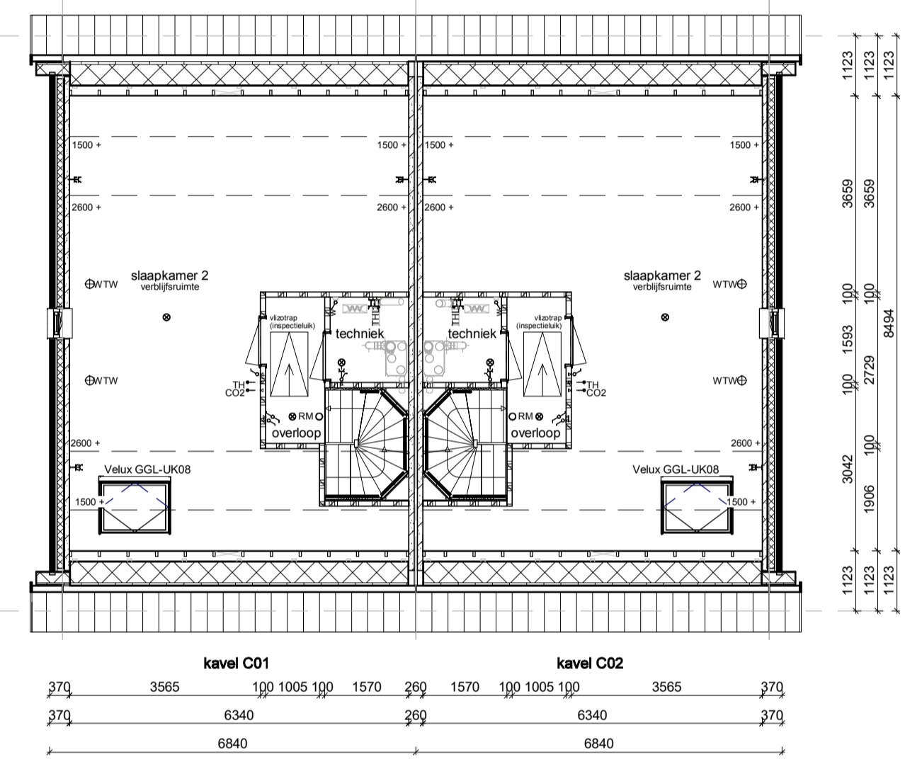
Verdieping
