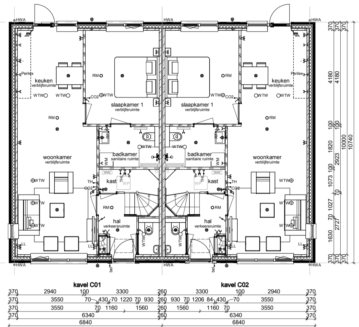
Begane grond
