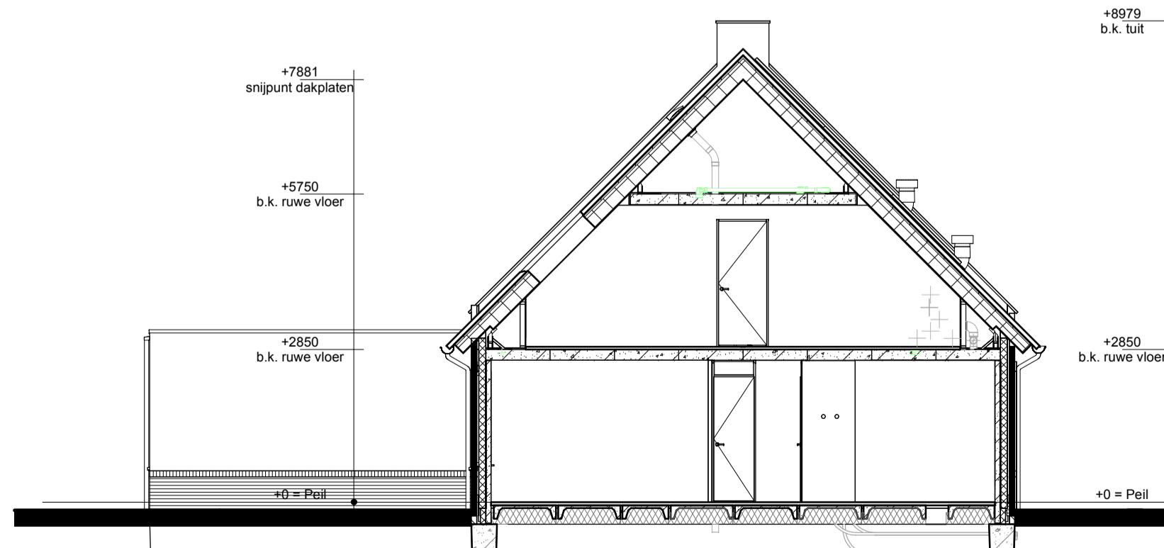
Doorsnede A1-A1
