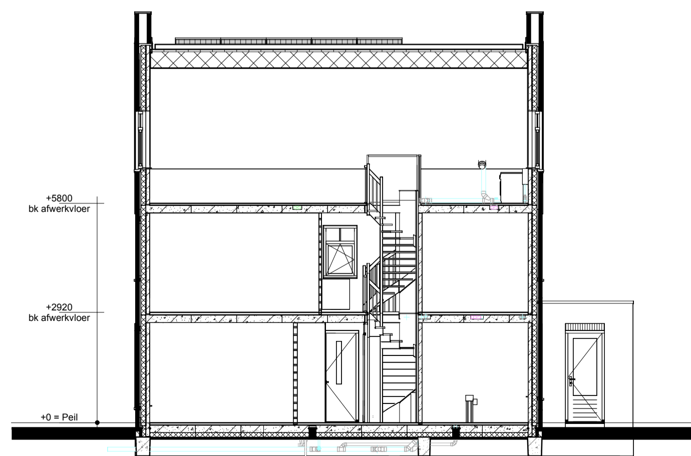
Doorsnede A5 - A5
