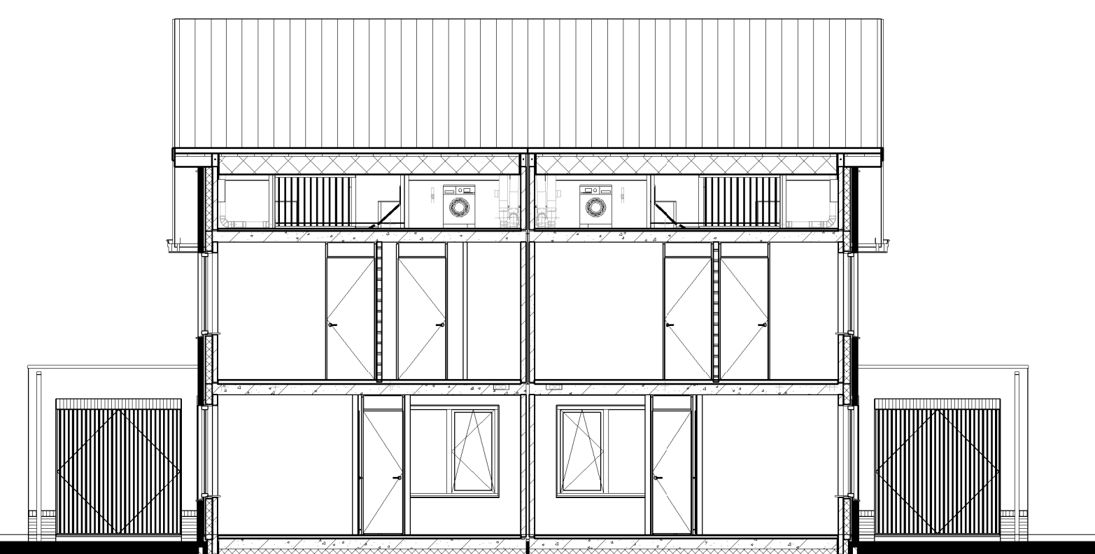
Doorsnede B2-B2
