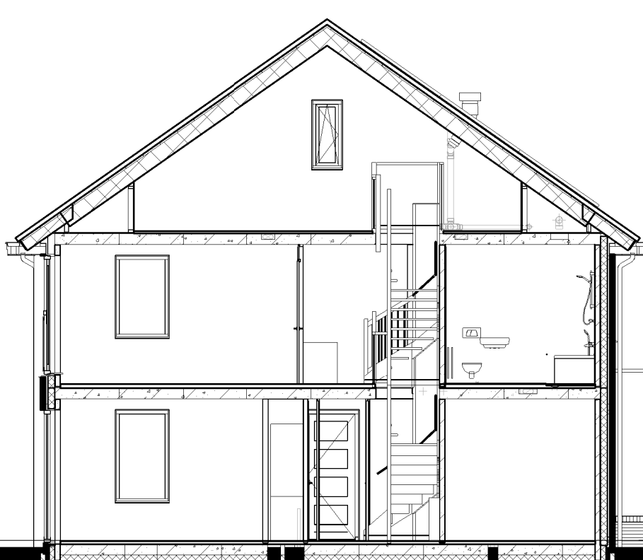
Doorsnede A2-A2
