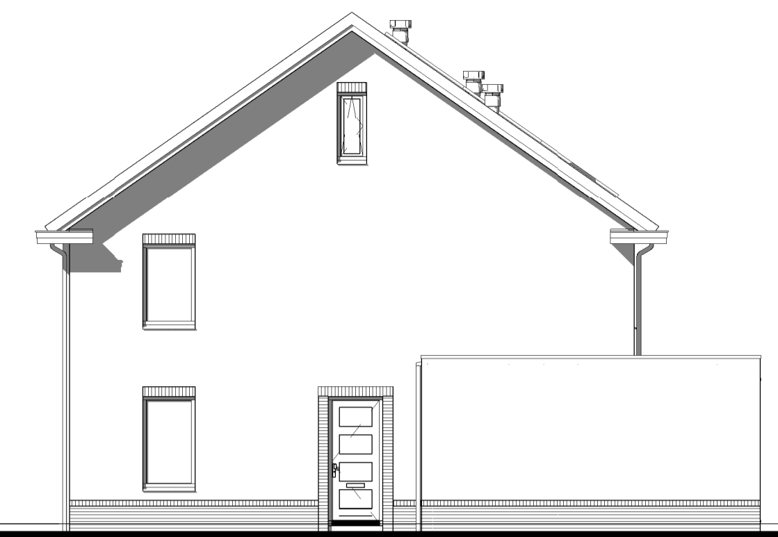
Rechter zijgevel
