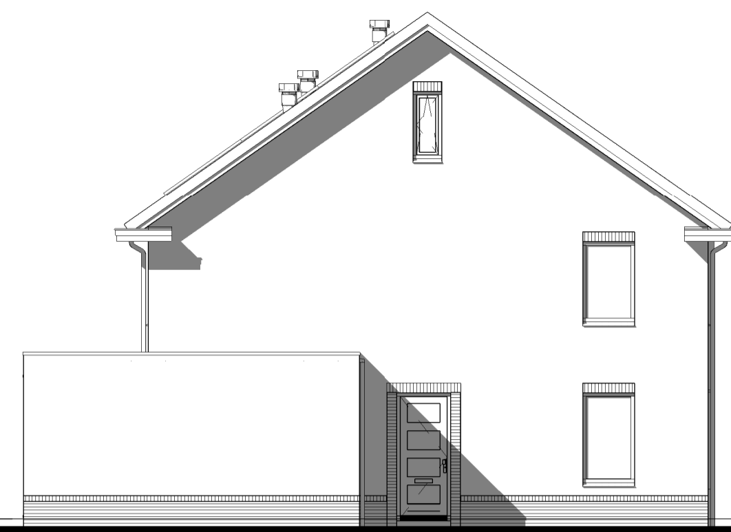
Linker zijgevel
