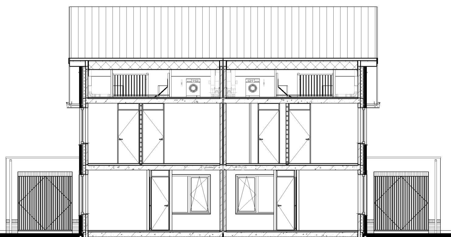
Doorsnede B3-B3
