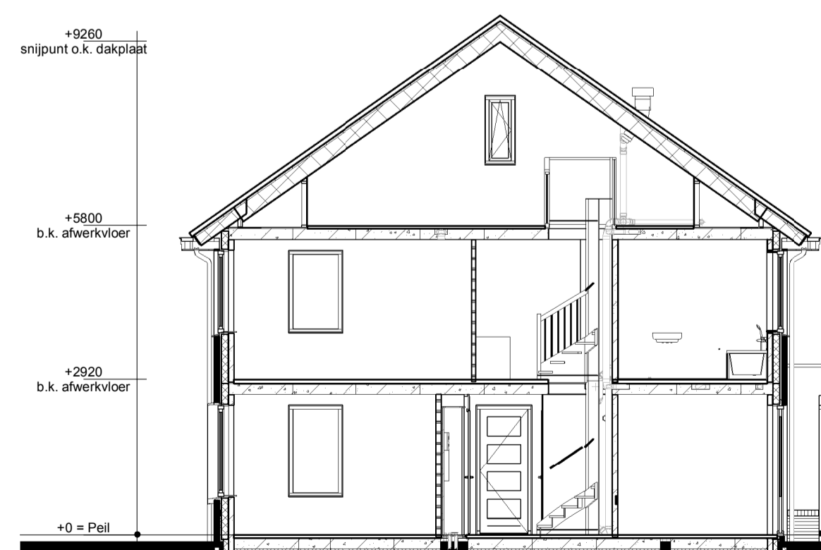
Doorsnede A3-A3
