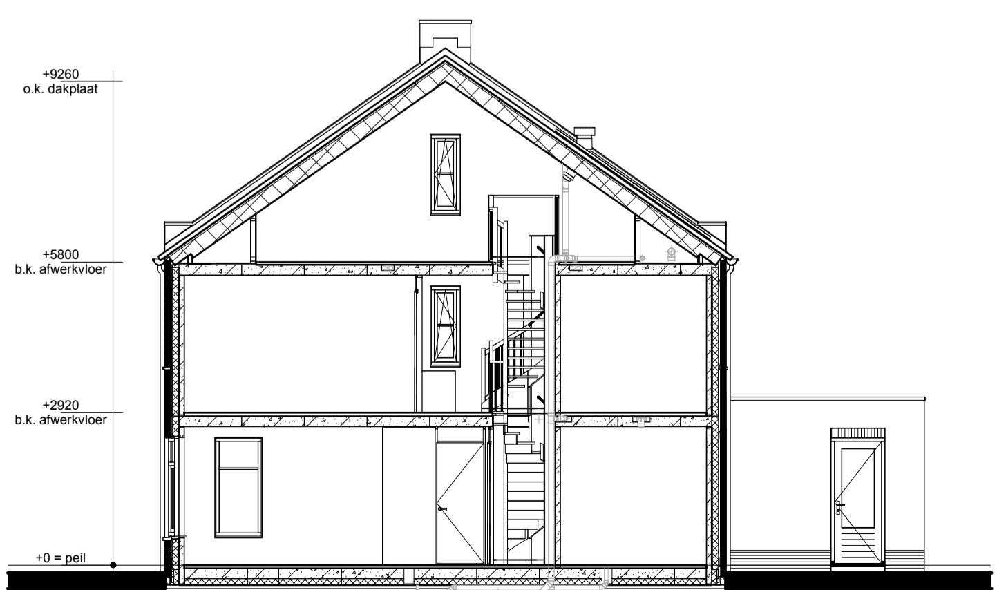
Doorsnede A6-A6
