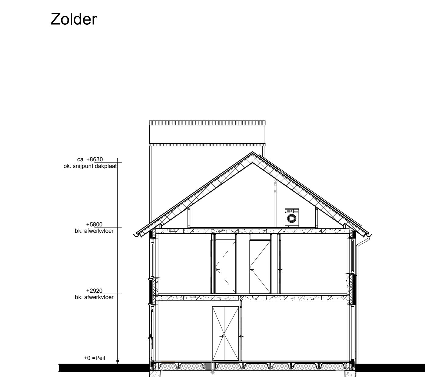
Doorsnede A1-A1
