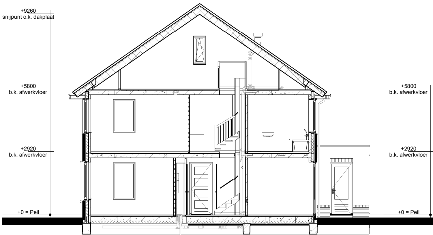
Doorsnede A5-A5
