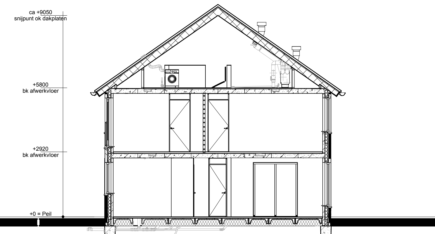
Doorsnede A2-A2
