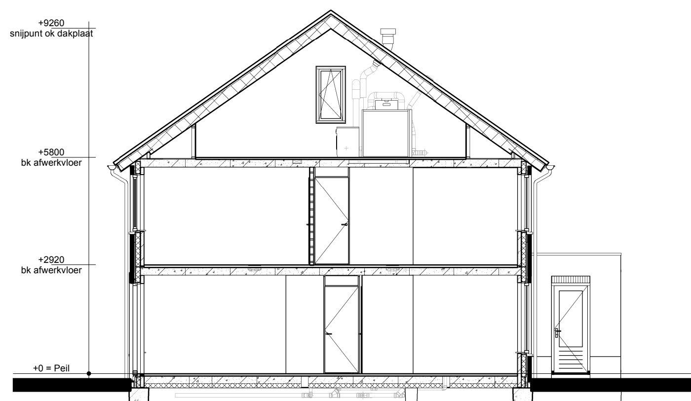
Doorsnede A1-A1
