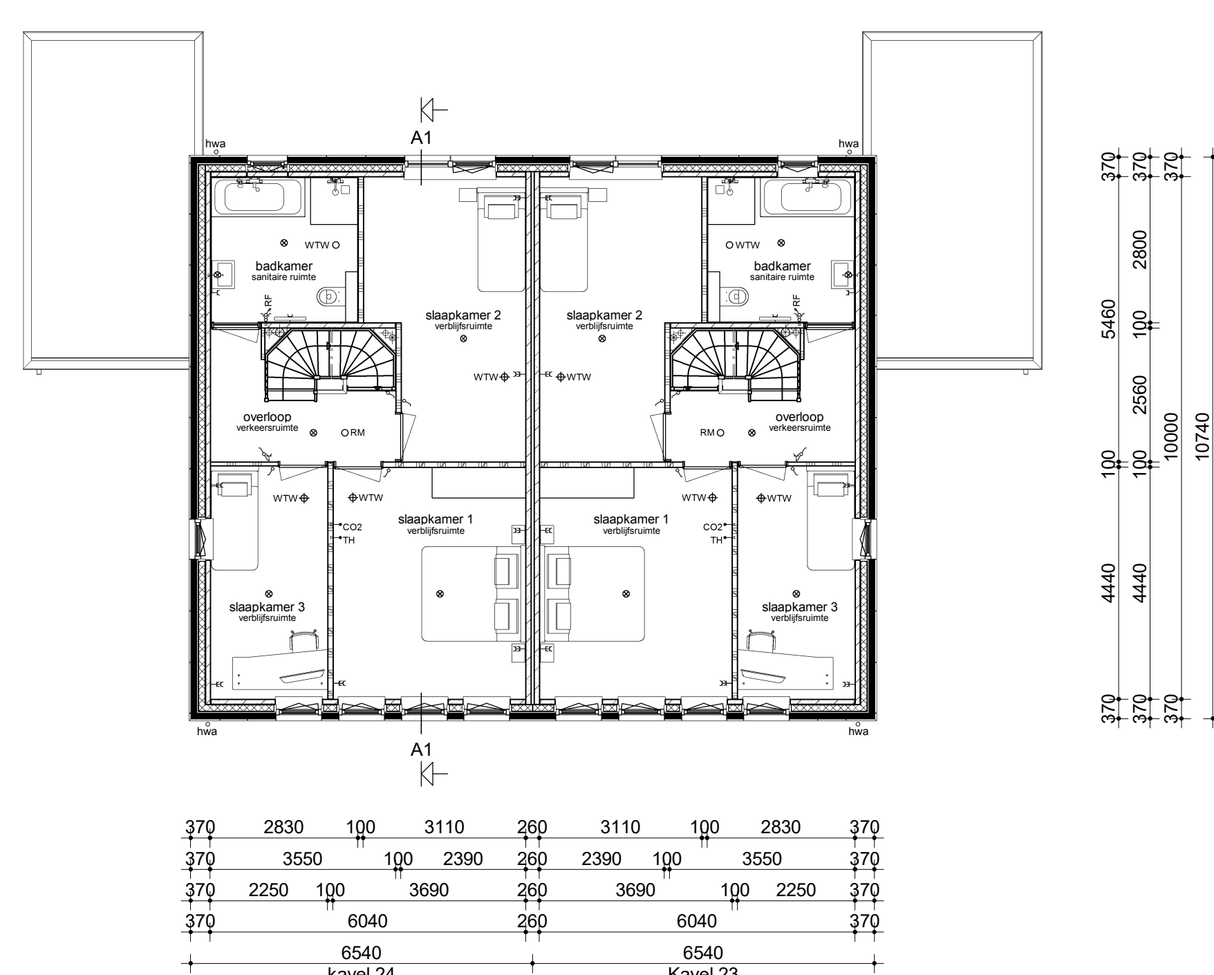
Verdieping
