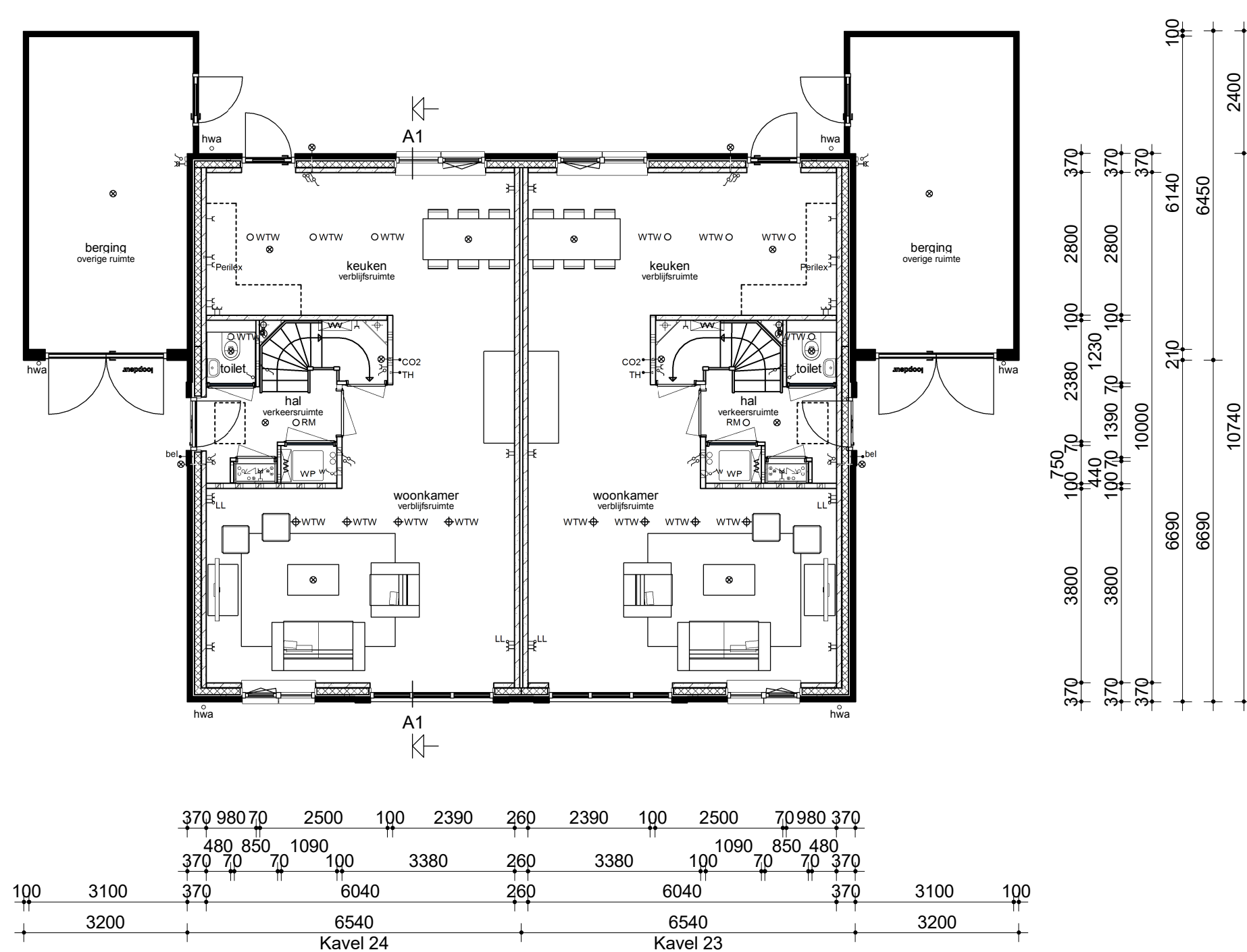
Begane grond
