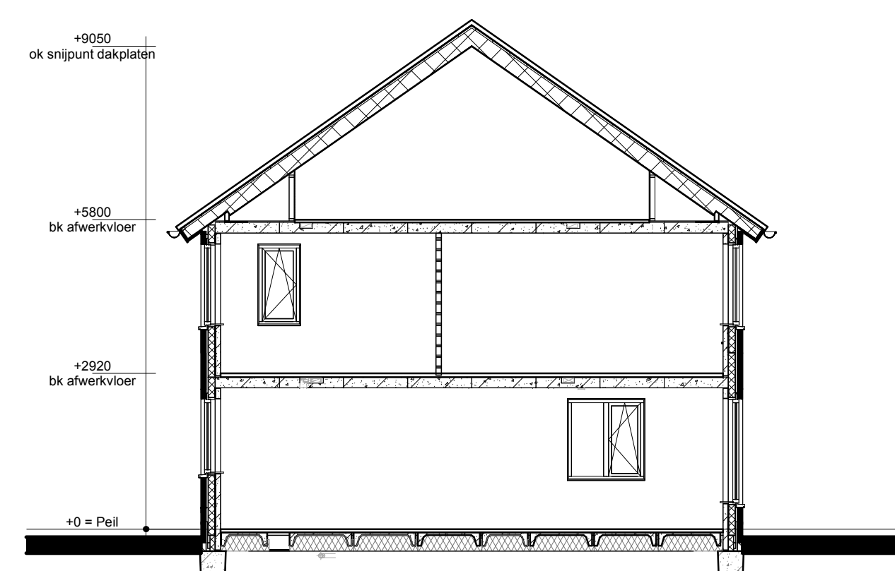
Doorsnede A1-A1
