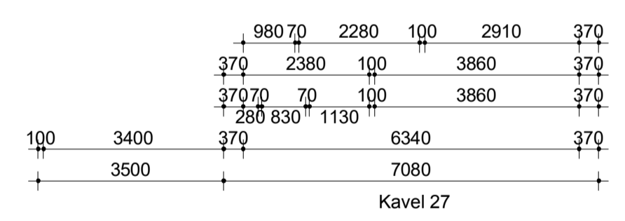
Begane grond
