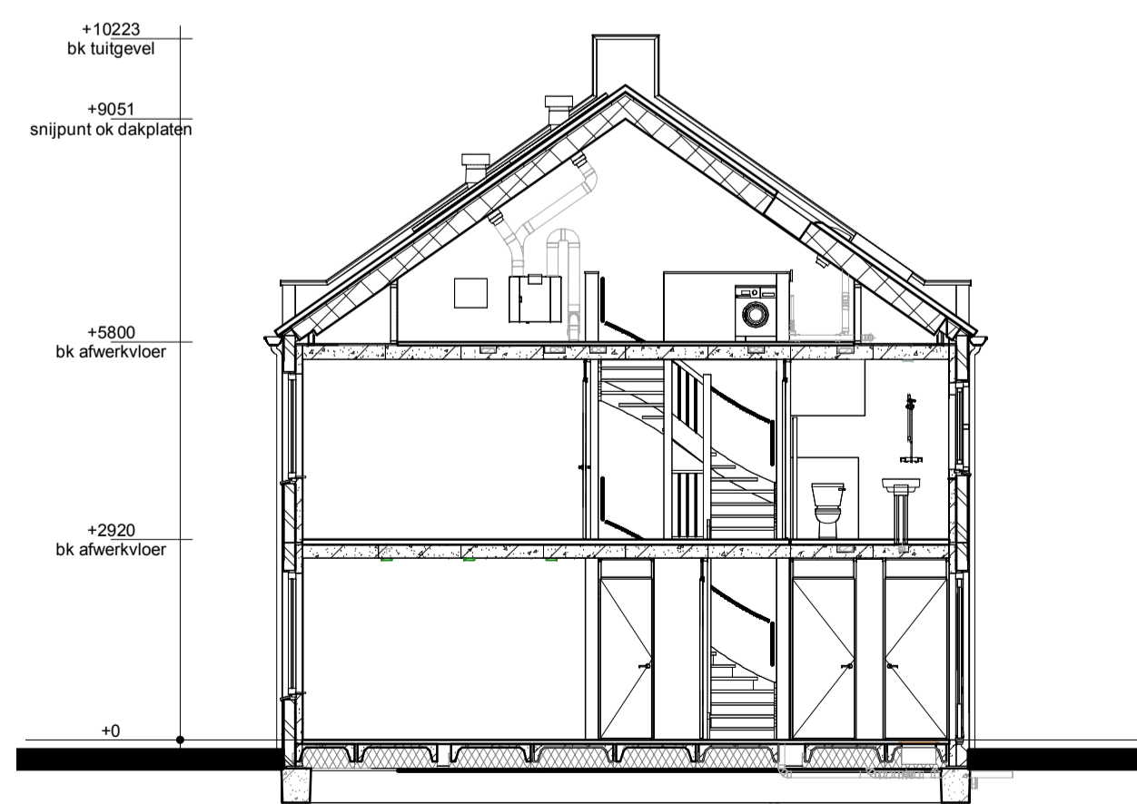
Doorsnede AA
