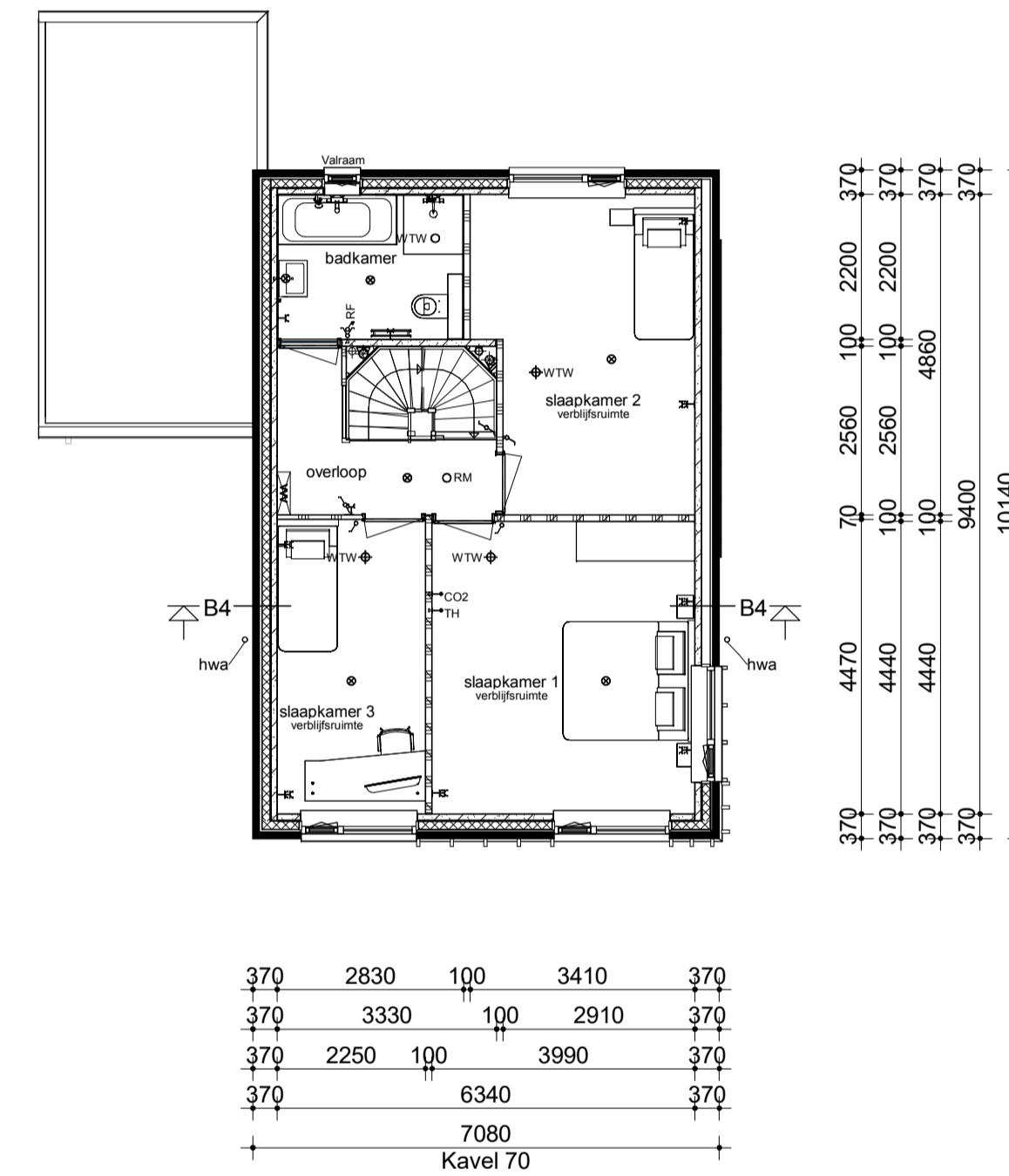
Verdieping
