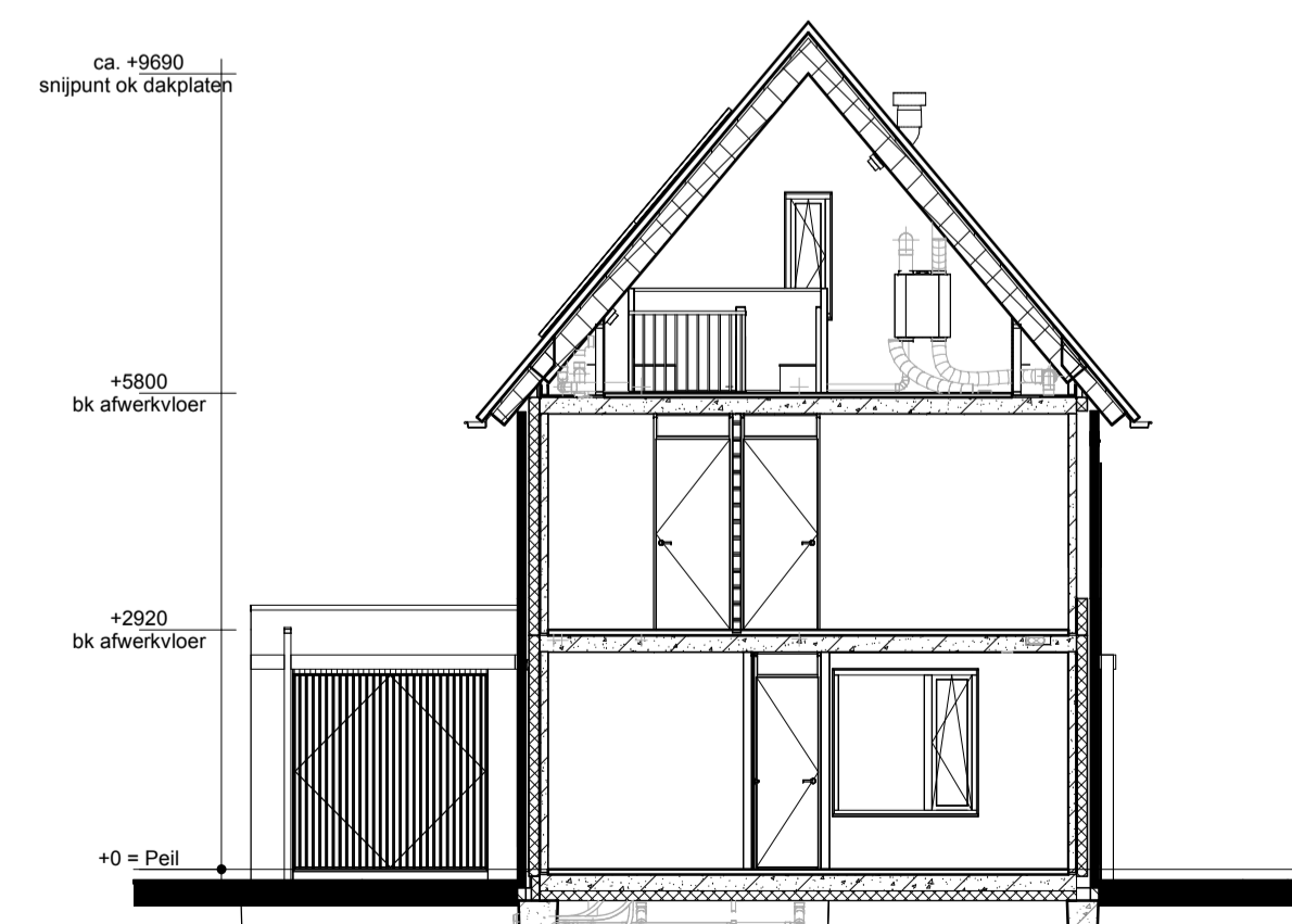
Doorsnede B4
